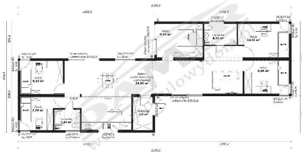
Rzut modułu typ „Z” 131,67 m 2 wersja z aneksem kuchennym człony 1
